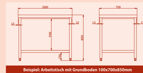
Beispiel: Arbeitstisch mit Grundboden 100x700x850mm
